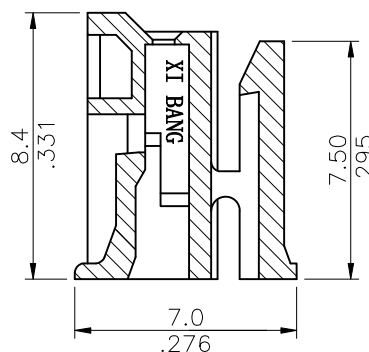
A-A SEC.
