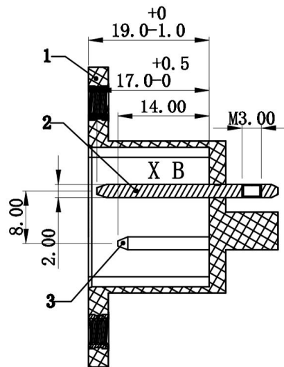
剖面 A-A
