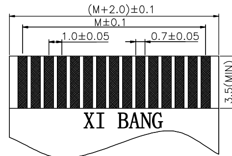
适用FPC寸法 APPLICABLE FPC
