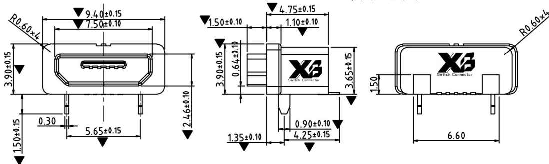
组装示意图
