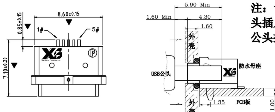
组装示意图
