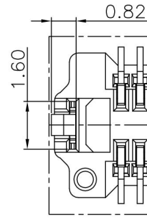
DETAIL B 2:1
