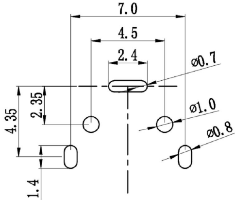
PCB线路板安装图(±0.1)
