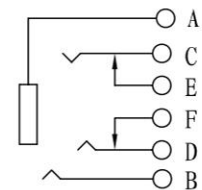
ST-053A SCHEMATIC
