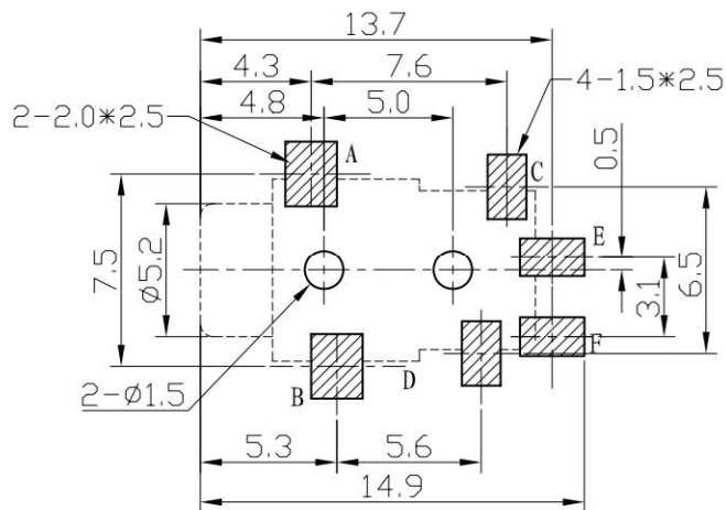
P.C.B LAYOUT
