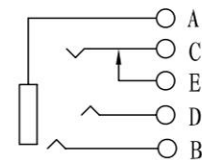
ST-053C SCHEMATIC
