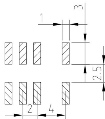
P.C.B LAYOUT
