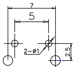
安装孔位图
