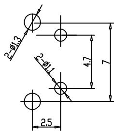
安装孔位图
