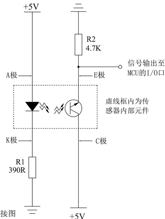
电路图
