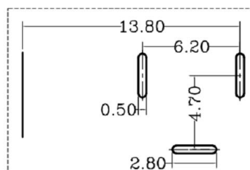
印刷电路板焊接处尺寸图 印刷电路板厚度T=1.60mm
