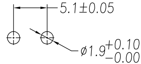
PCB开孔尺寸
