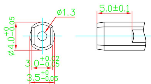
推柄局部尺寸详图
