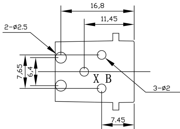
线路板按装尺寸示意图
