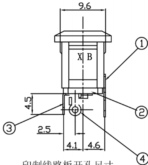
印制线路板开孔尺寸
