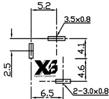
印制线路板开孔尺寸
