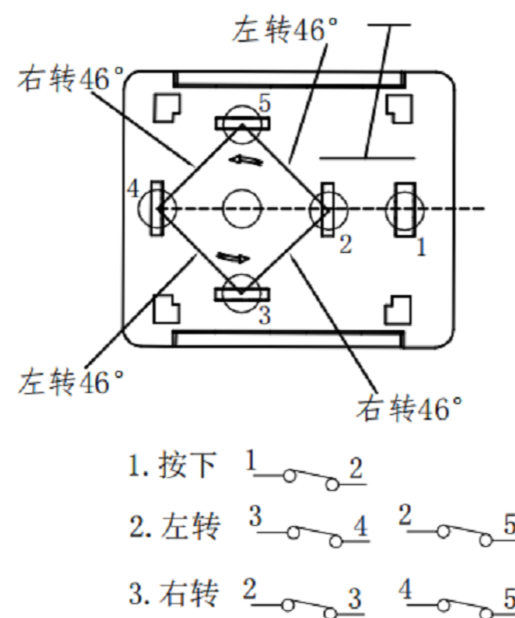
电原理图
