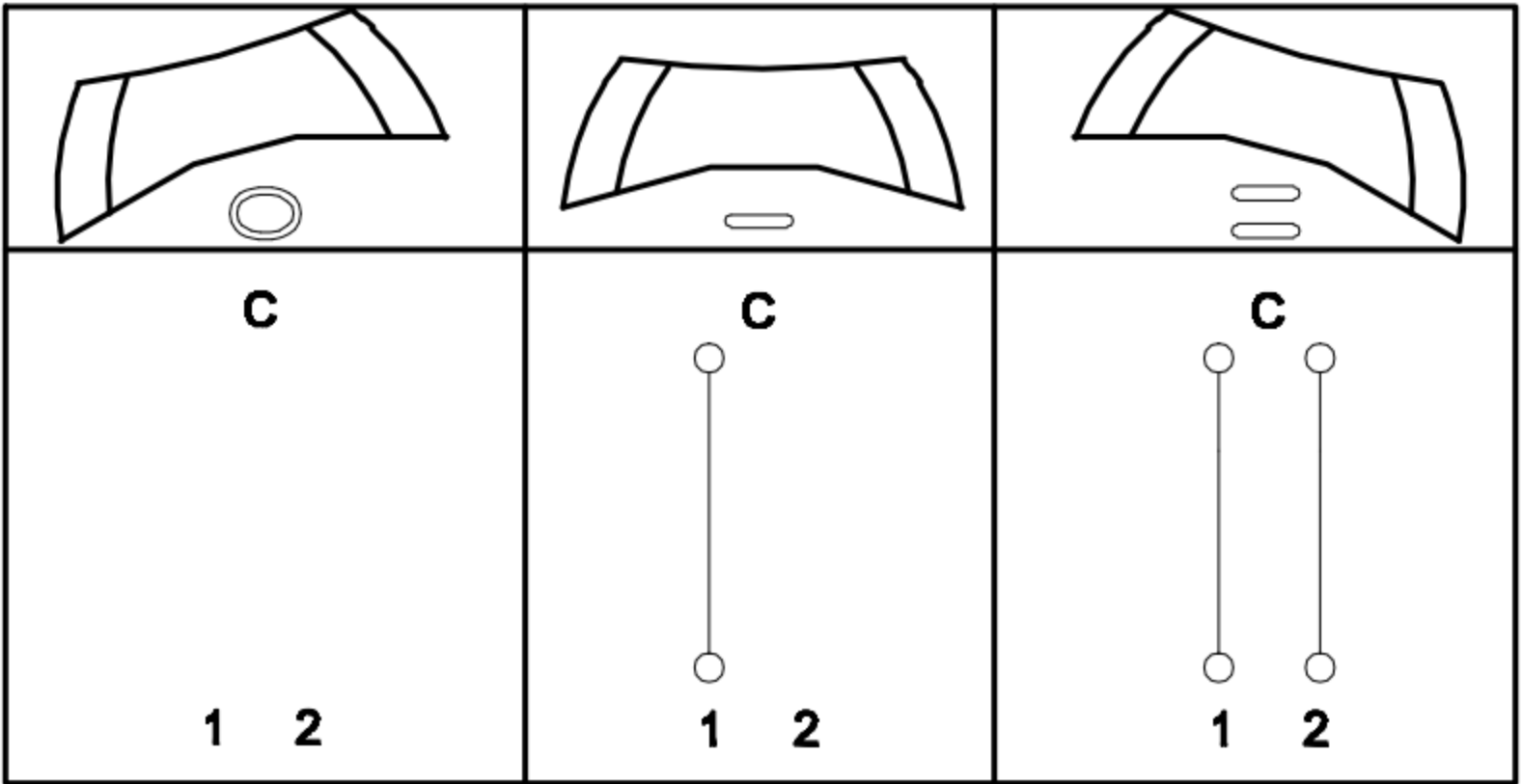
线路/ Circuit
