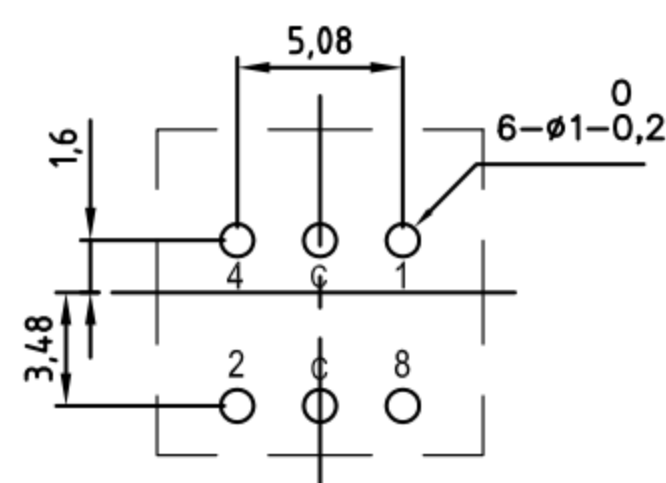
P.C.B. LAYOUT
