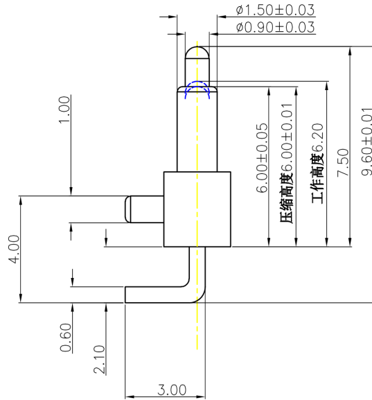
图为焊盘位置和大小
