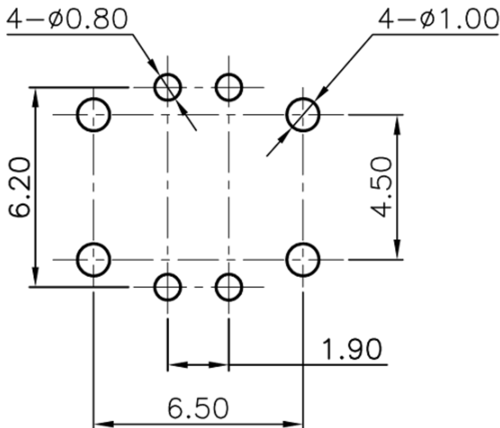
P.C.B LAYOUT
