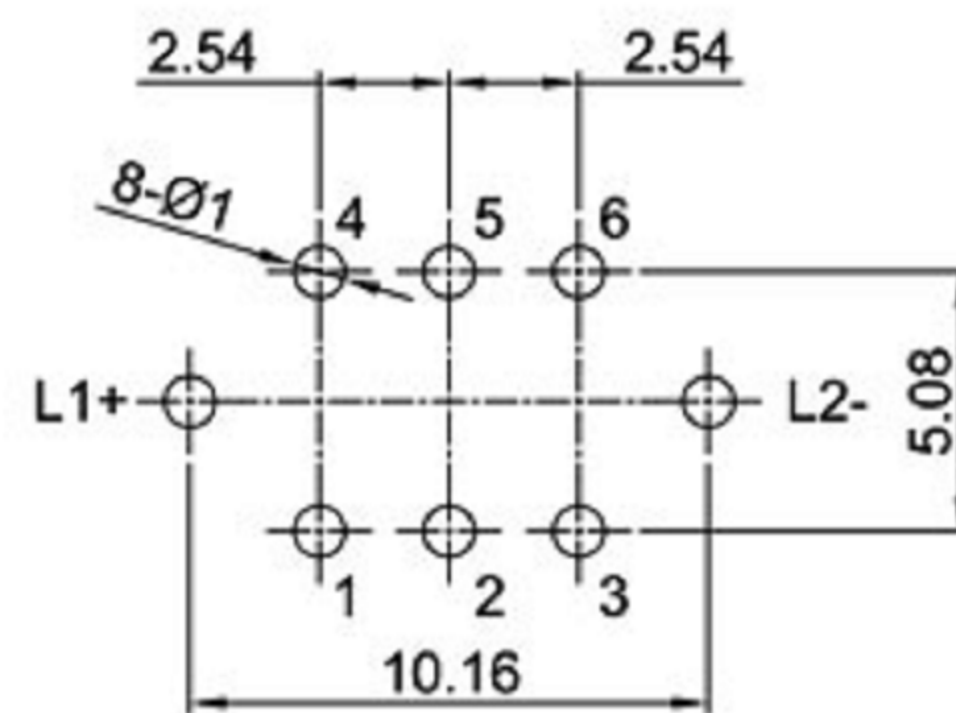
P.C.B. LAYOUT
