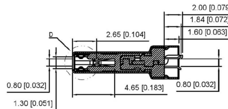
SECT A-A
