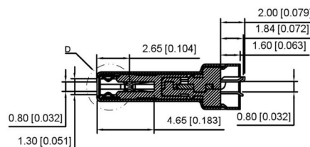
SECT A-A
