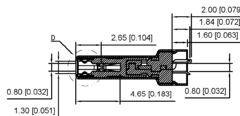
SECT A-A
