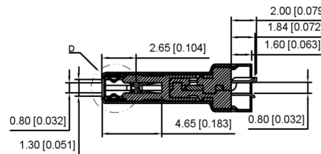
SECT A-A
