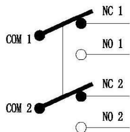
电路图 双联单控
