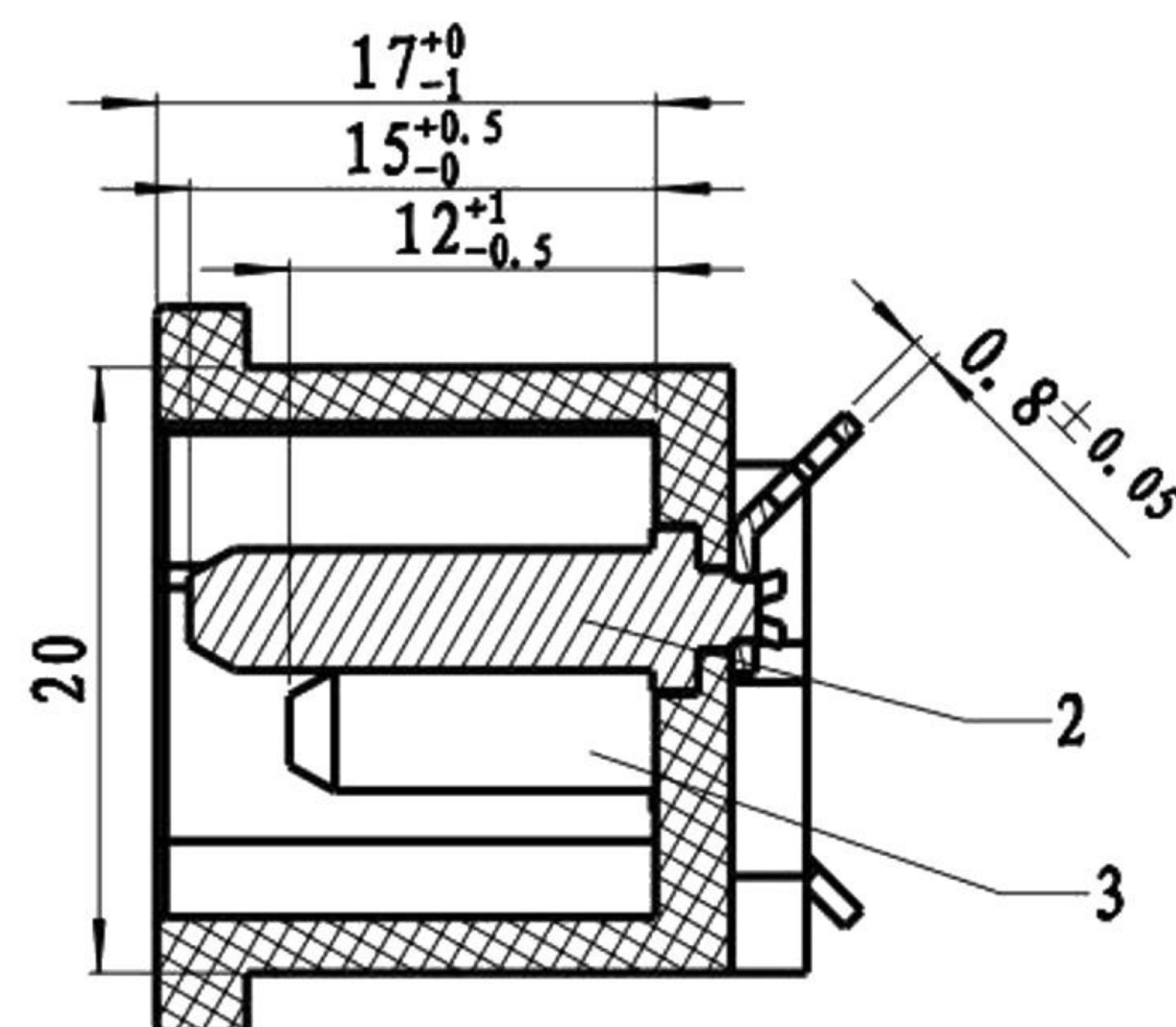
剖面 A-A
