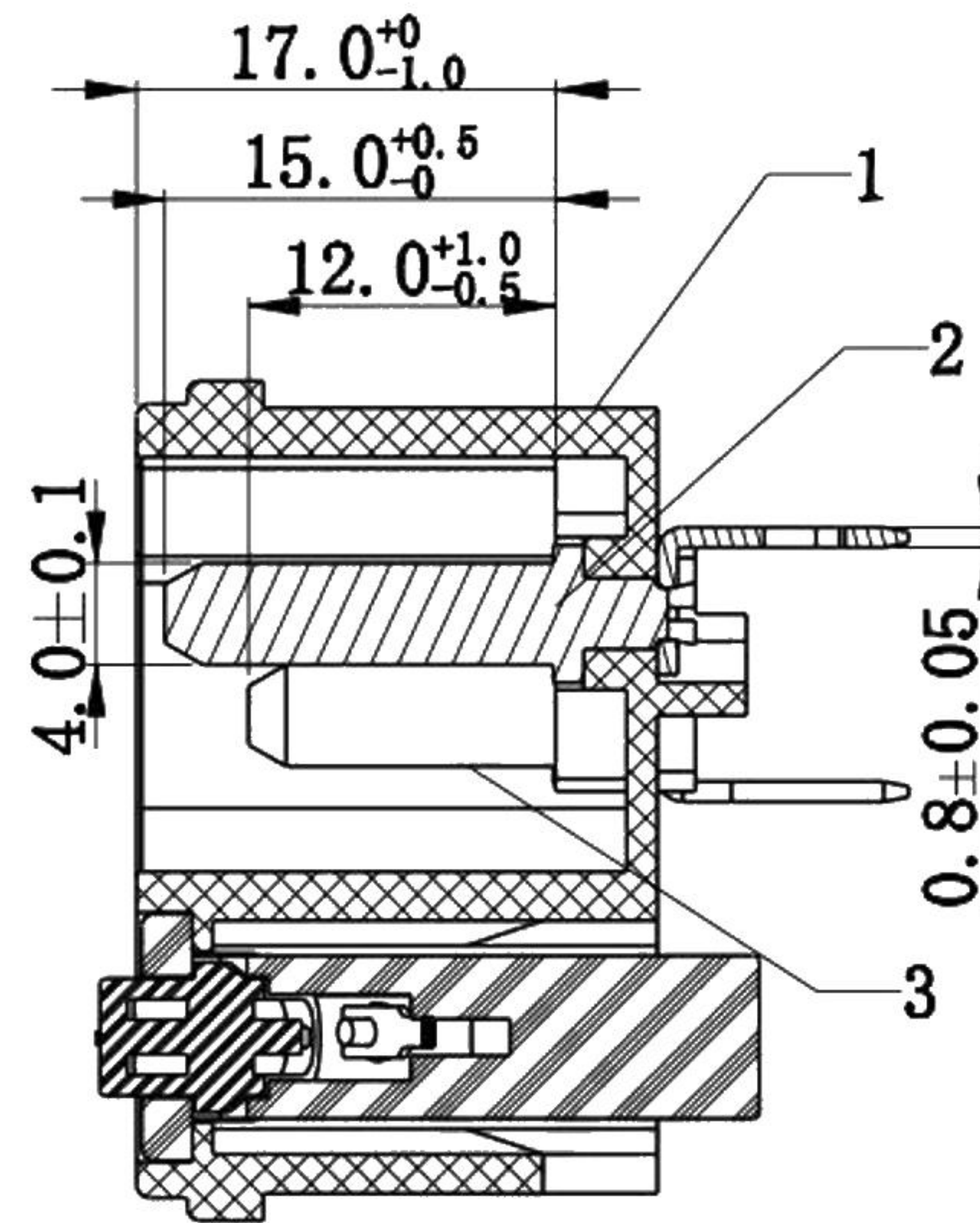
剖面 A-A
