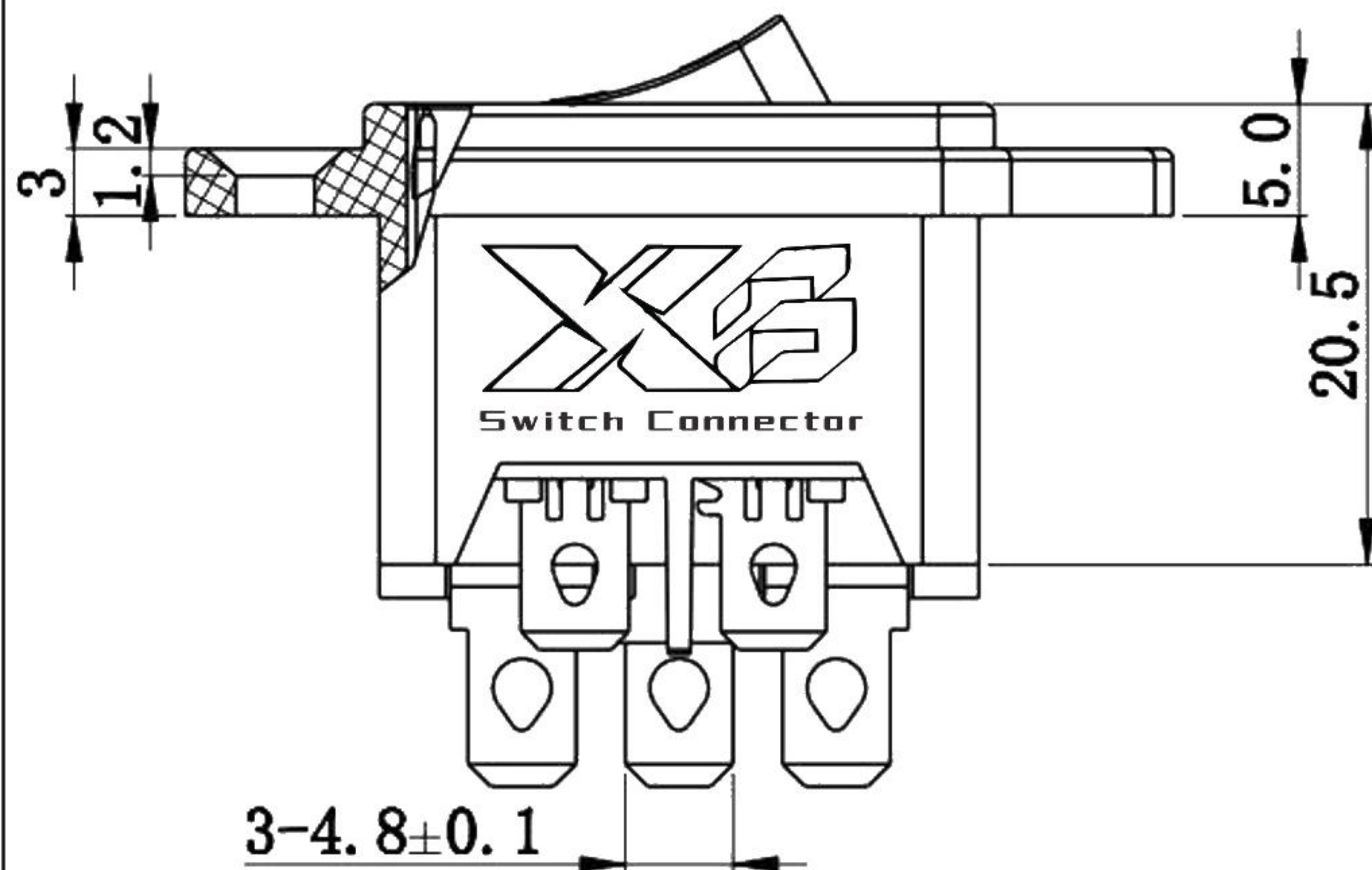
剖面 B-B
