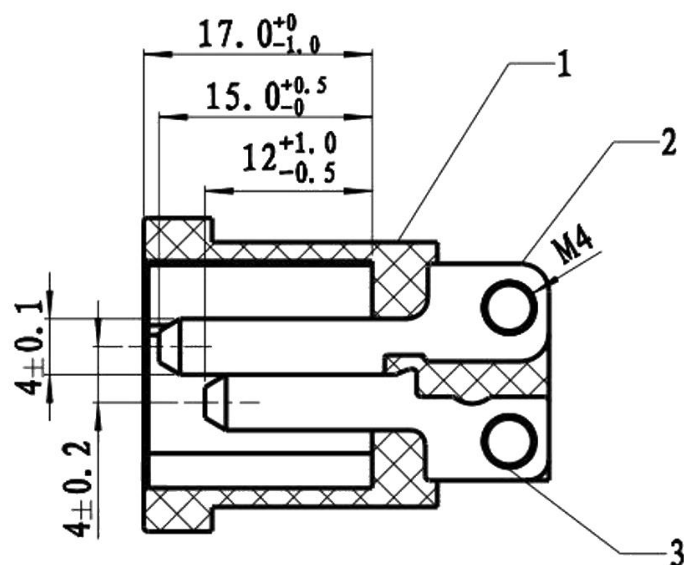
剖面 A-A
