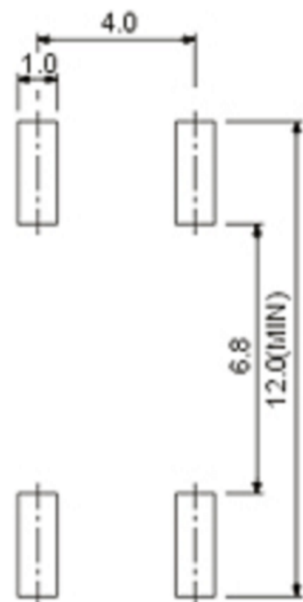
P.C.B LAND DIMENSION
