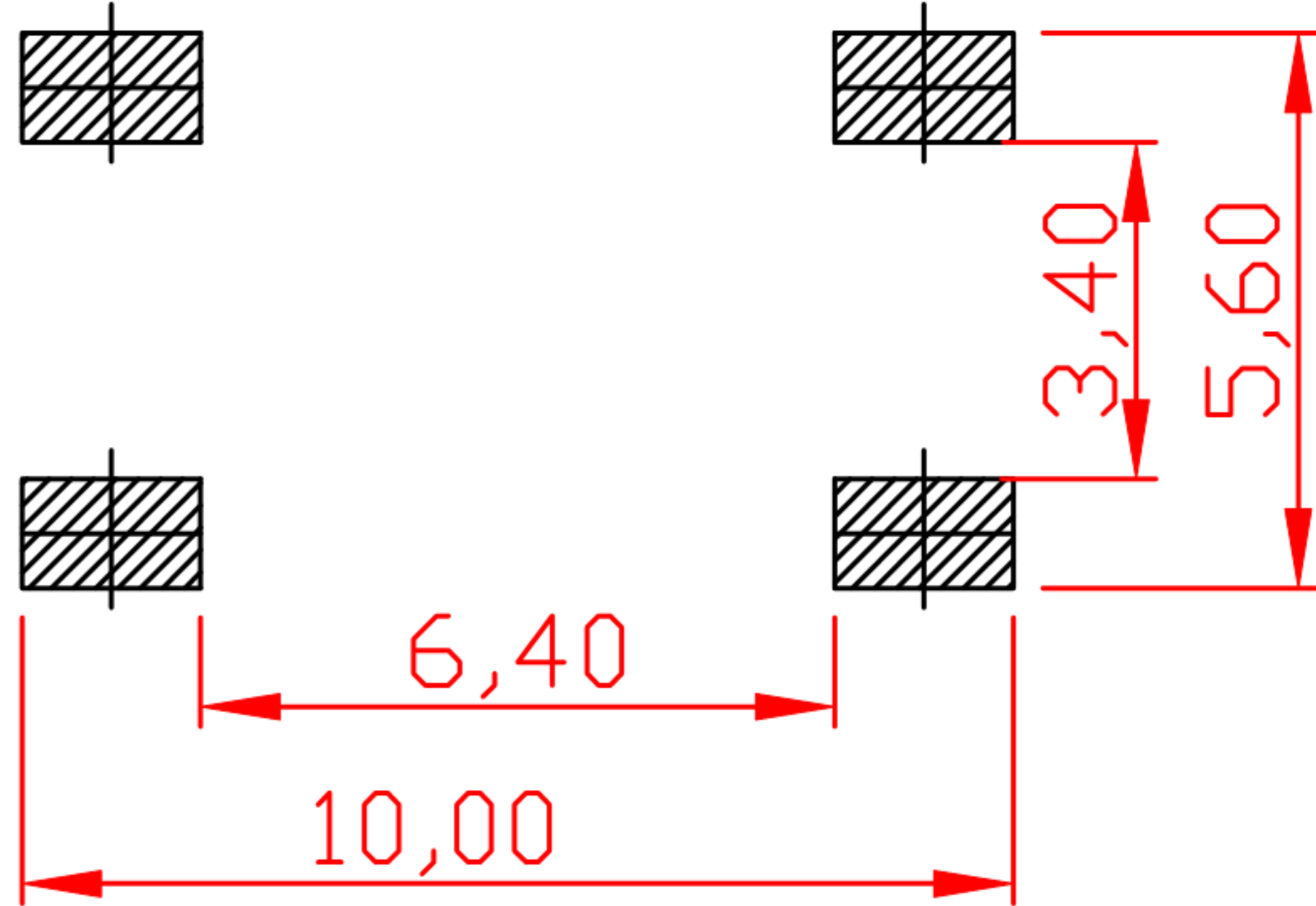
PCB. 焊接图
