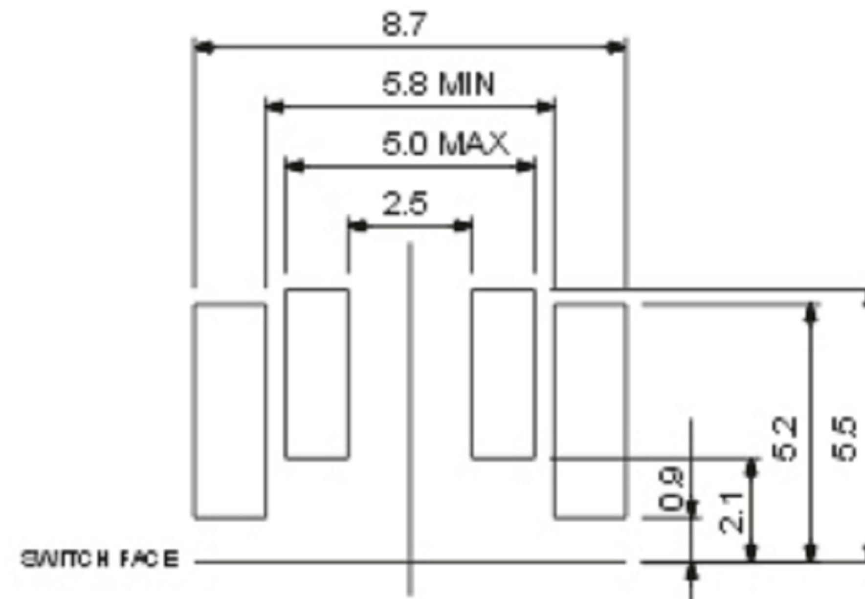
P.C.B LAND DIMENSION
