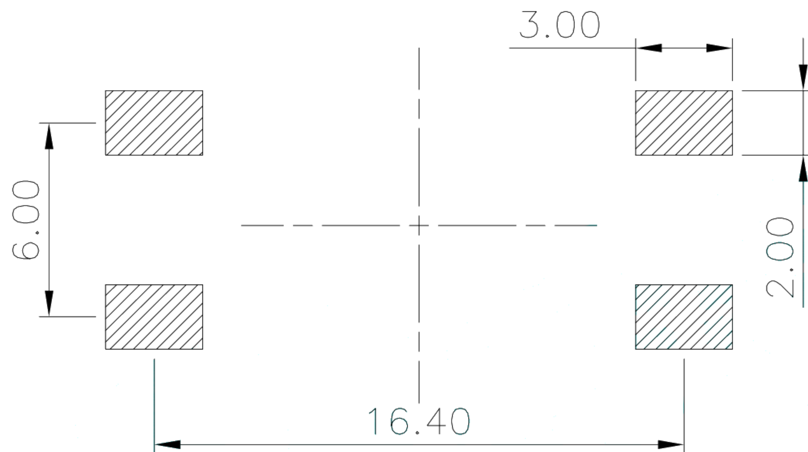
PCB Layout(Pattern side)
