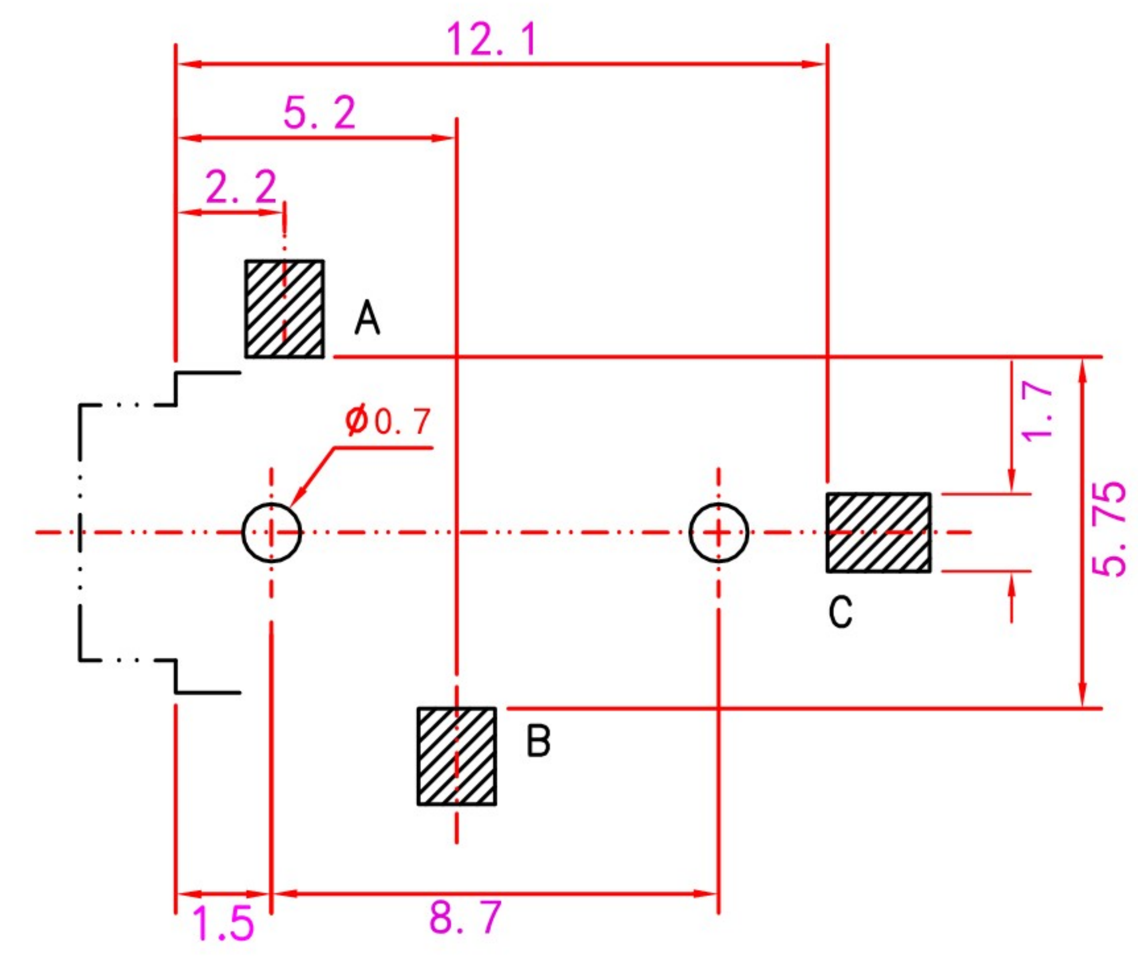
印制板开孔示意图
