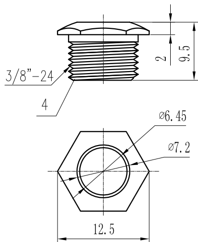
铜套
