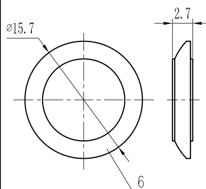
垫片2
