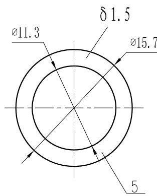
垫片1
