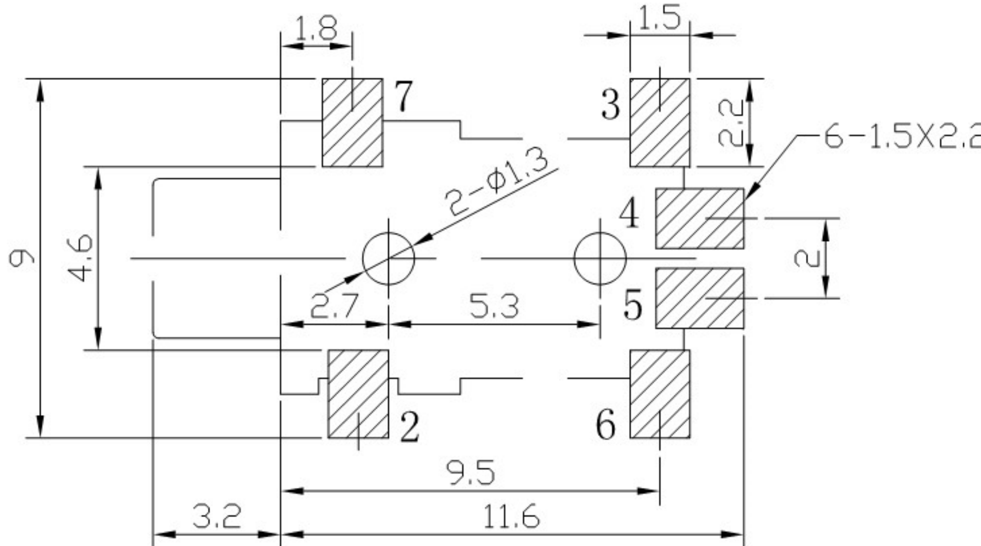
线路板开孔尺寸 TOP VIEW
