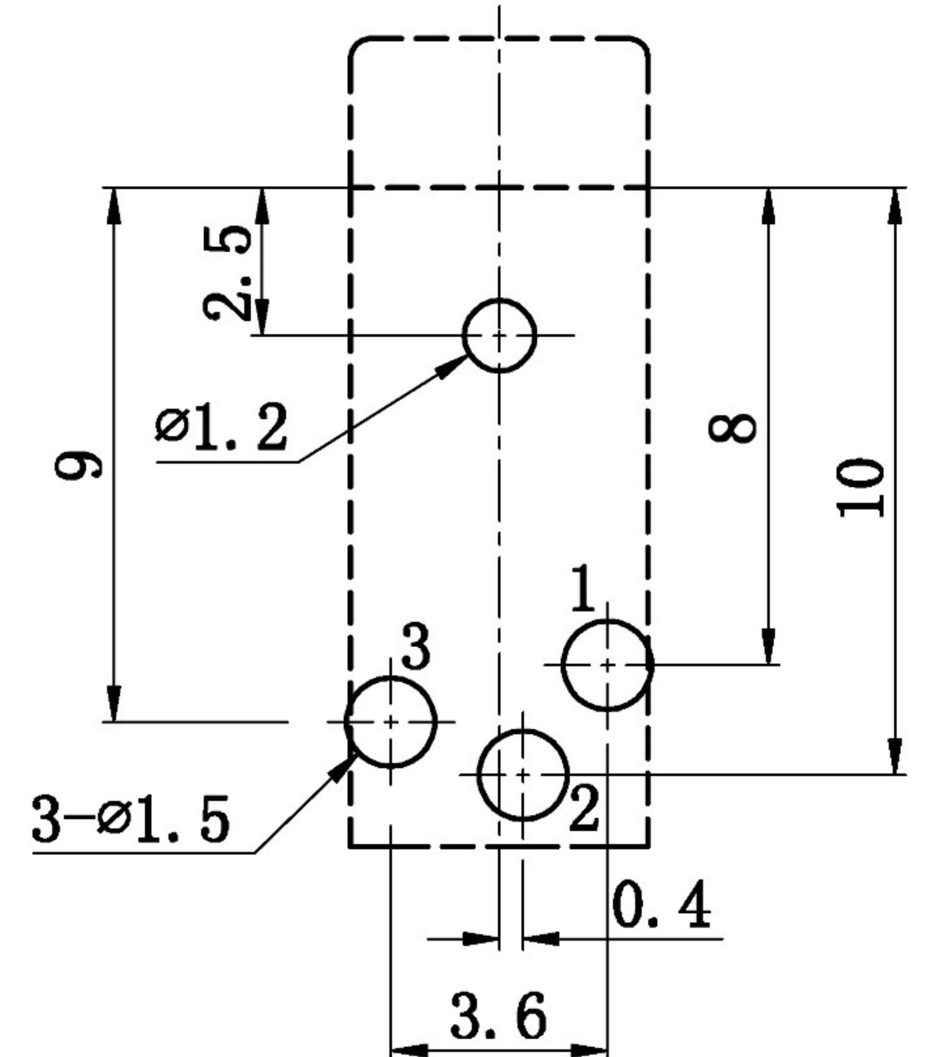
线路板开孔尺寸 TOP VIEW
