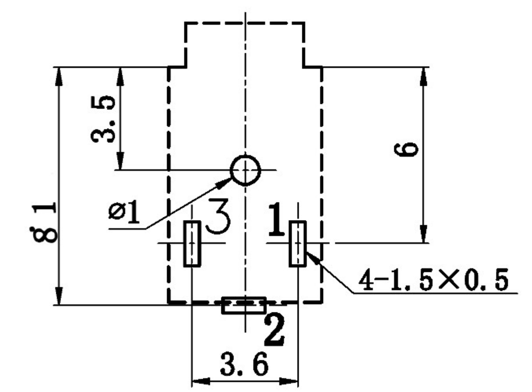
线路板开孔尺寸 (顶 视)
