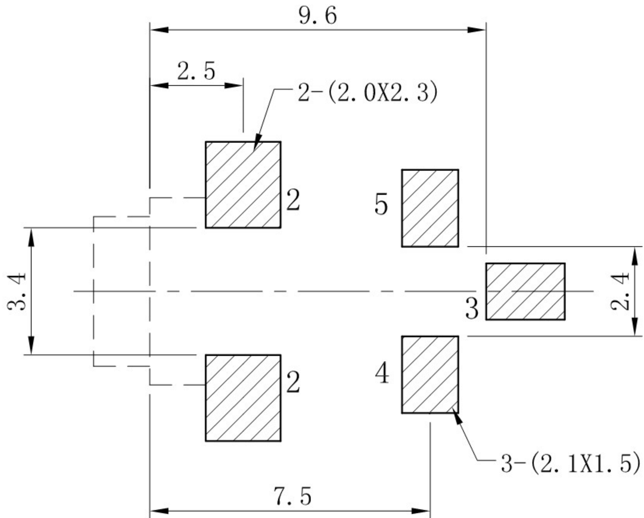
线路板开孔尺寸 P.C.B LAYOUT
