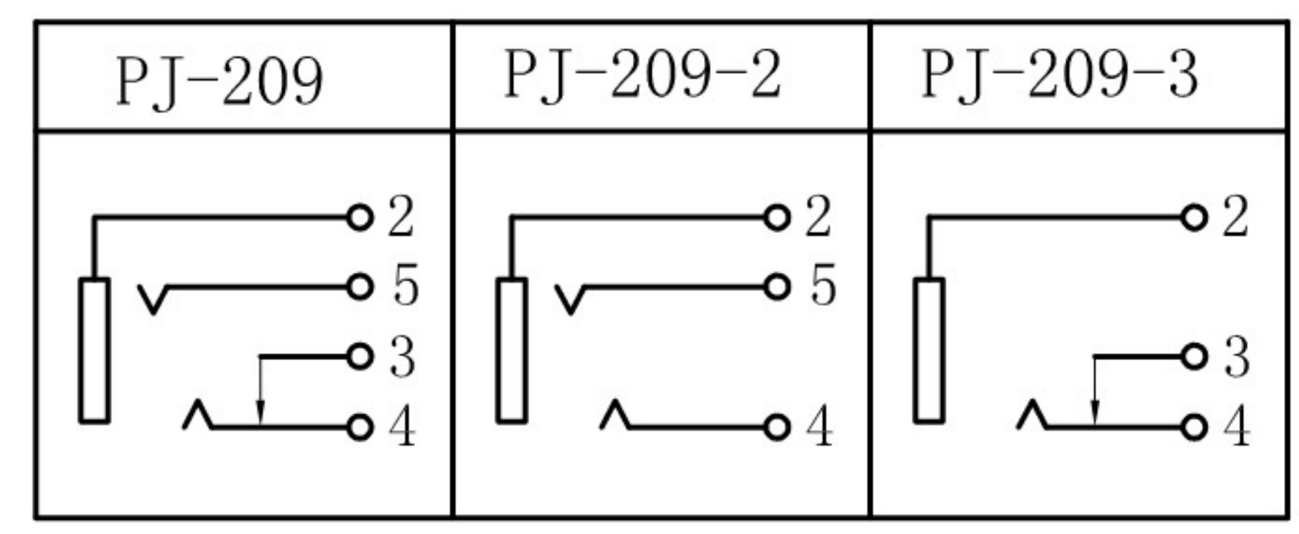
按点示意图 SCHEMATIC
