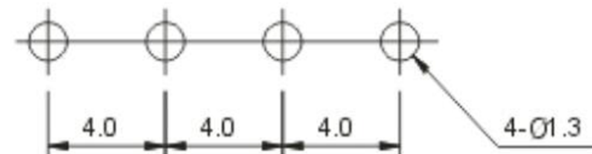
P.C.B HOLE DIMENSION
