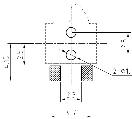
印制电路板及焊接安装孔参考图 (自A方向看)
