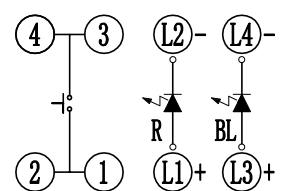
电原理图
