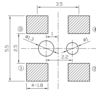
安装位置图
