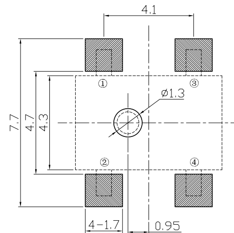
安装尺寸图
