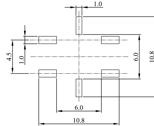
P.C.B. LAYOUT
