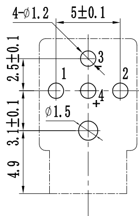
元件面孔位图
