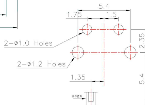
PCB Layout(Pattern side) Scale: 1 : 2
