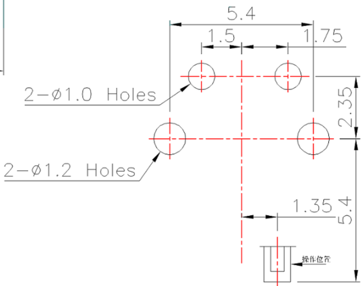
PCB Layout(Pattern side) Scale: 1 : 2
