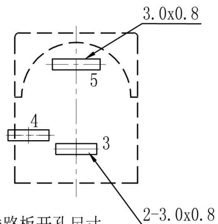
线路板开孔尺寸
